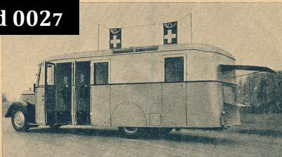
Automobil-Telephonsprechstationen — Bureau téléphonique automobile Ufficio telefonico-automobile
